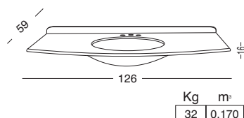
FH-INTV TOP INTEGRATO "SILICIUM GLASS" CON ALZATINA SAGOMATA INTEGRATED SILICIUM GLASS TOP WITH BACKSPLASH СТОЛЕШНИЦА СИЛИЦИУМ ГЛАСС ИТЕГРИРОВАННАЯ С ПРИСТЕННОЙ ПЛАНКОЙ
